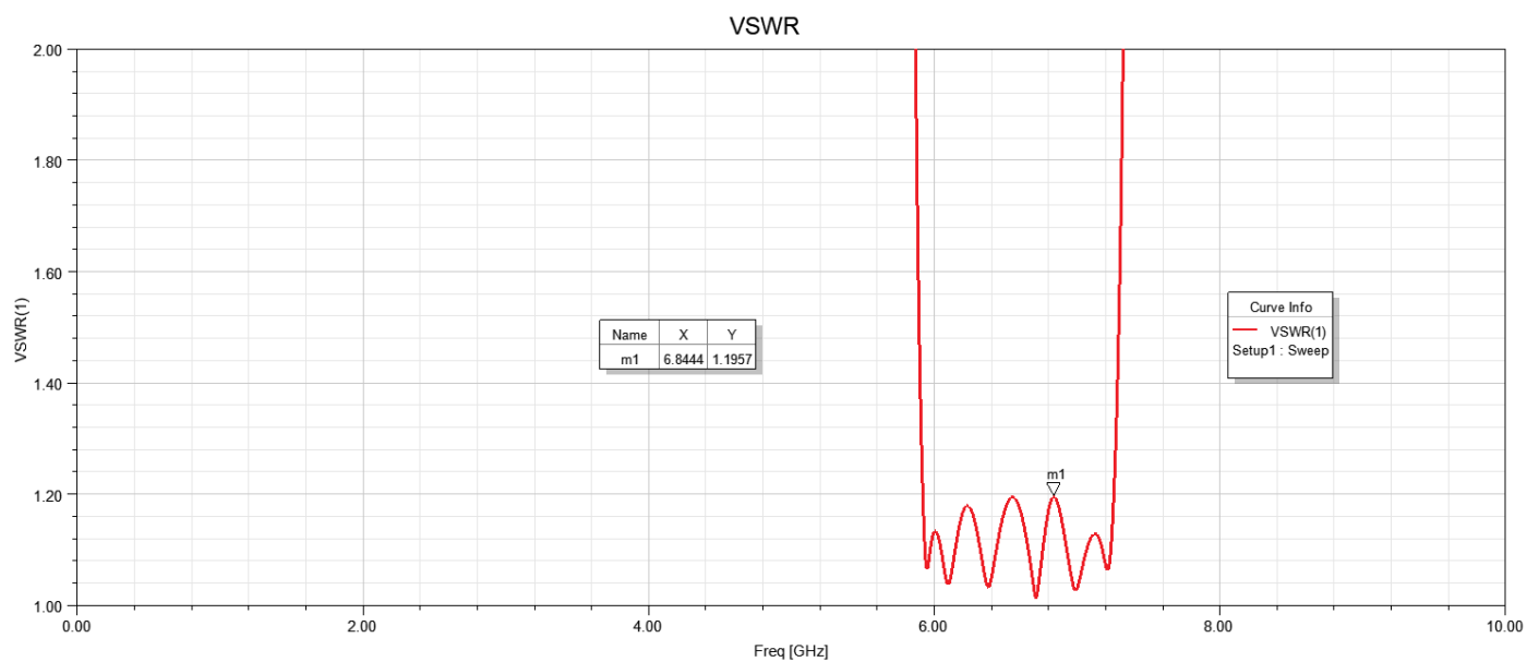
VSWR
