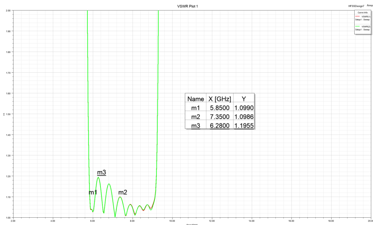
VSWR
