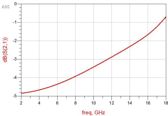
dB(S(2,1))
