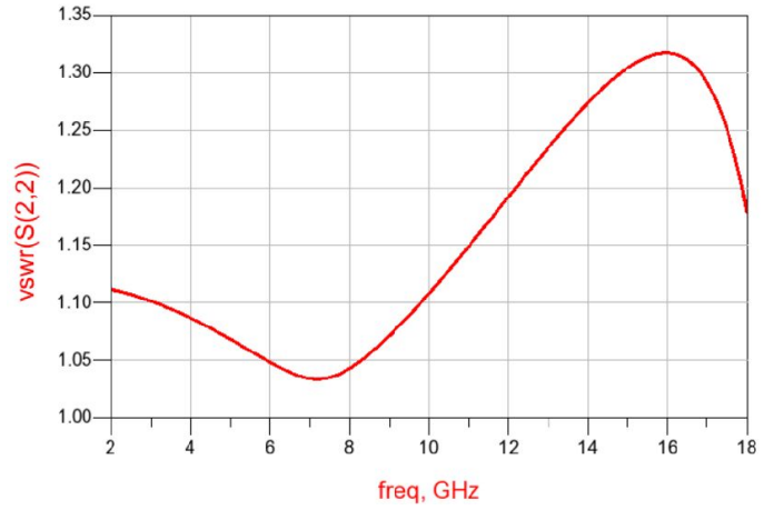
vswr(S(2,2))
